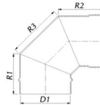
Koleno 90°
