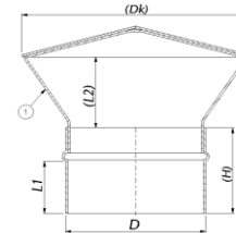
Strieška
