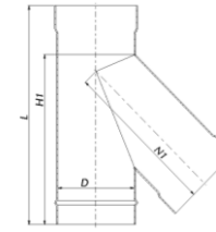
T-kus 45°
