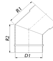
Koleno 45°
