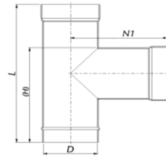
T-kus 90°
